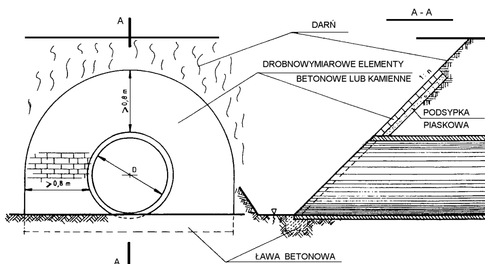
Rys. 2. Przykład umocnienia skarpy przy wlocie przepustu za pomocą drobnowymiarowych elementów z betonowej kostki brukowej lub kamienia
