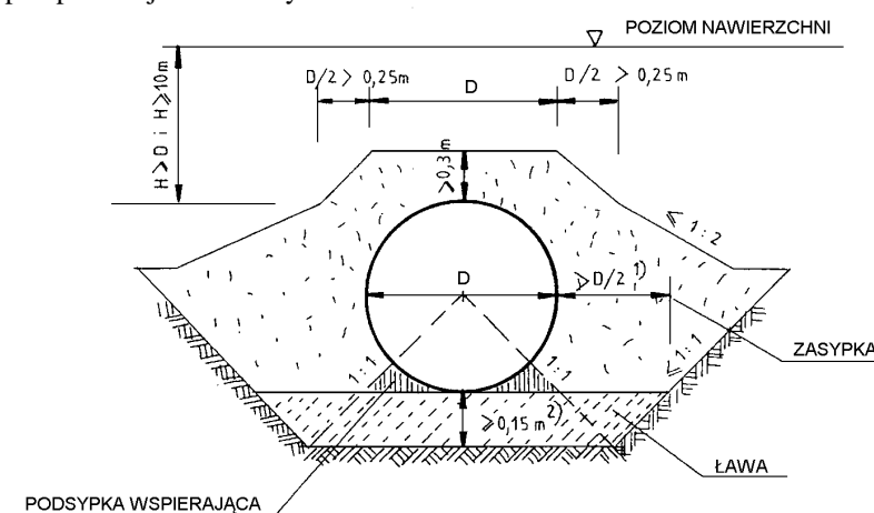
Rys. 1. Zasyпка nad przepustem jednorurowym
